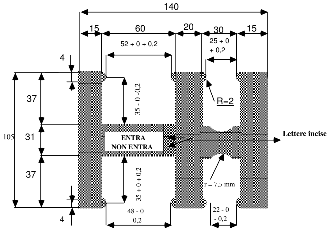
DIMA DI CONTROLLO DEGLI SPESSORI DELLA DERIVA
