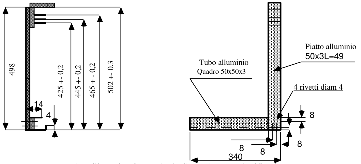
DIMA DI CONTROLLO DELLA LARGHEZZA E DELLA POSIZIONE DEI PUNTI DI CONTROLLO DELLO SPESSORE DELLA DERIVA
